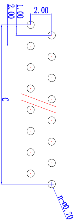
1.0-A-nPW 印制电路板 P.C.B Layout
